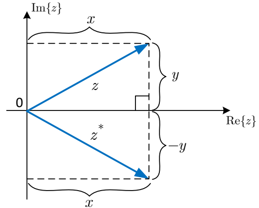
Σχήμα 1.2: Ζεύγος συζυγών μιγαδικών z, z^* .
