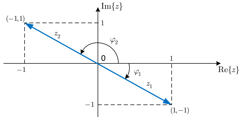
Σχήμα 1.6: Μιγαδικοί z_1 και z_2 .
