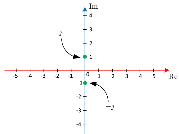
Σχήμα 1.1: Μιγαδικό επίπεδο.
