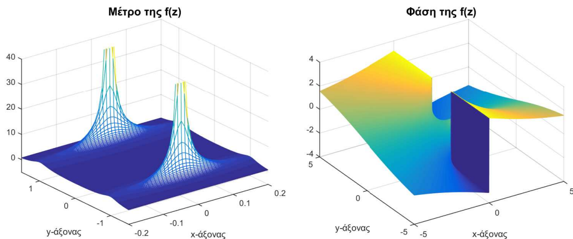
Σχήμα 1.11: Μέτρο και Φάση της συνάρτησης Παραδείγματος 1.8.
