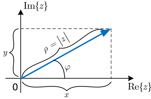
Σχήμα 1.4: Πολική μορφή μιγαδικού αριθμού z .
