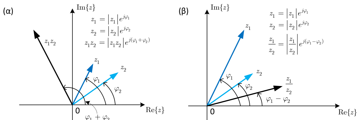
Σχήμα 1.8: (α) Πολλαπλασιασμός και (β) διαίρεση μιγαδικών αριθμών στο μιγαδικό επίπεδο.
