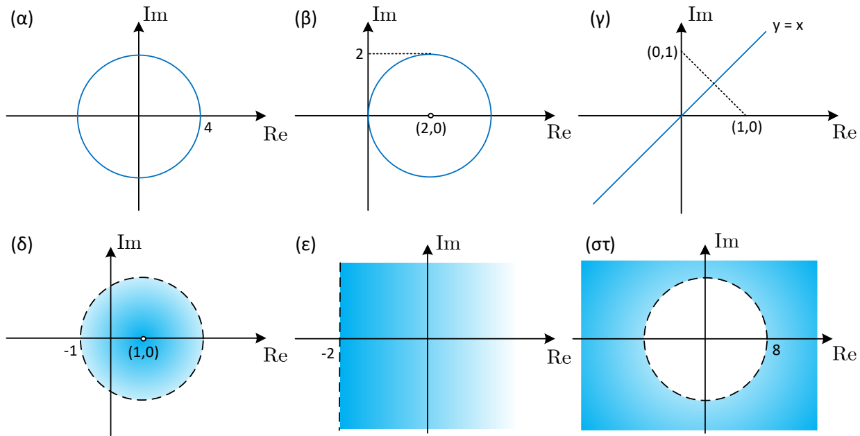
Σχήμα 1.9: Γεωμετρικοί τόποι Παραδείγματος 1.7.
