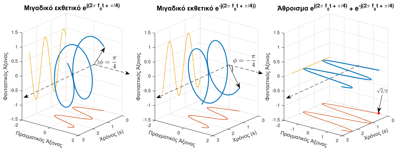
Σχήμα 1.14: Συζυγείς μιγαδικές εκθετικές συναρτήσεις με αρχική φάση \phi = \pi/4 και το πραγματικό άθροισμά τους. Το περιστρεφόμενο διάνυσμα (με μαύρο χρώμα) βρίσκεται σε τυχαία θέση του άξονα του χρόνου (διακεκομμένη μαύρη γραμμή)
