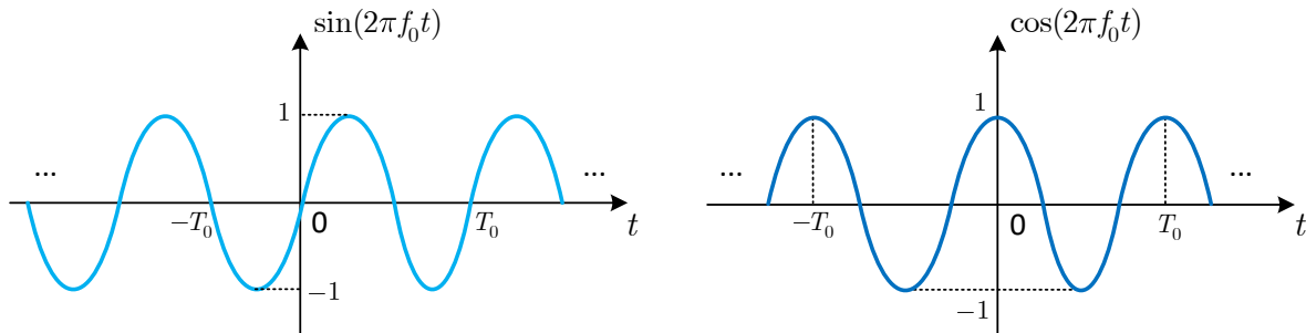
Σχήμα 1.15: Ημίτονο (αριστερά) και Συνημίτονο (δεξιά).
