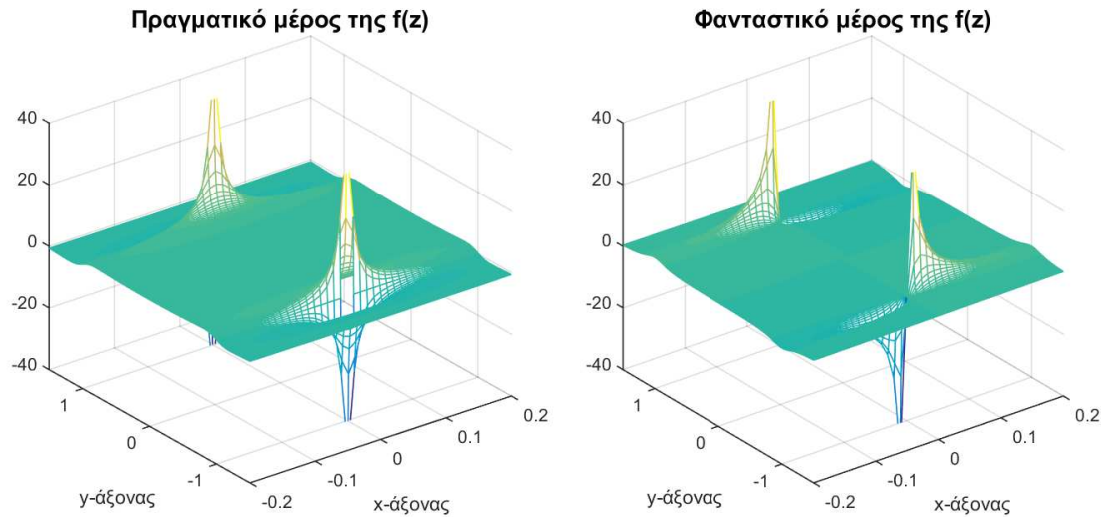
Σχήμα 1.10: Πραγματικό και Φανταστικό μέρος της συνάρτησης του Παραδείγματος 1.8.
