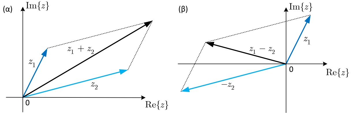
Σχήμα 1.3: (α) Πρόσθεση και (β) αφαίρεση μιγαδικών αριθμών στο μιγαδικό επίπεδο.
