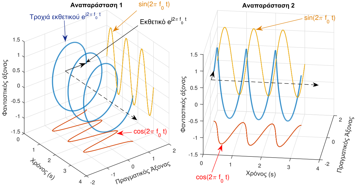
Σχήμα 1.12: Μιγαδική εκθετική συνάρτηση e^{j2\pi f_0 t} , μαζί με το πραγματικό και φανταστικό μέρος της, από δυο όψεις στον τριδιάστατο μιγαδικό χώρο.
