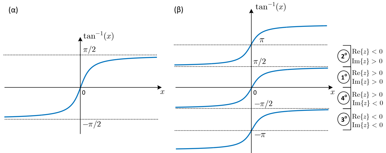
Σχήμα 1.5: (α) Πρωτεύουσα τιμή φάσης και (β) πρωτεύουσα και δευτερεύουσες τιμές φάσης.
