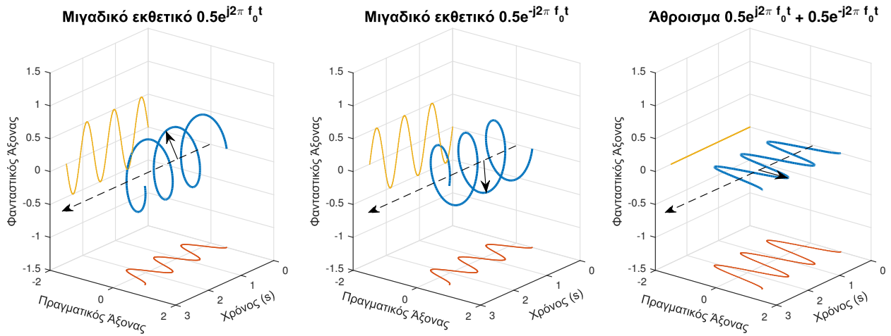
Σχήμα 1.13: Συζυγείς μιγαδικές εκθετικές συναρτήσεις και το πραγματικό άθροισμά τους. Το περιστρεφόμενο διάνυσμα (με μαύρο χρώμα) βρίσκεται σε τυχαία θέση του άξονα του χρόνου (διακεκομμένη μαύρη γραμμή).
