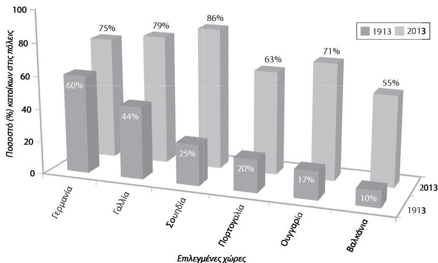
Διάγραμμα 0.1. Αστικοποίηση, 1913-2013
